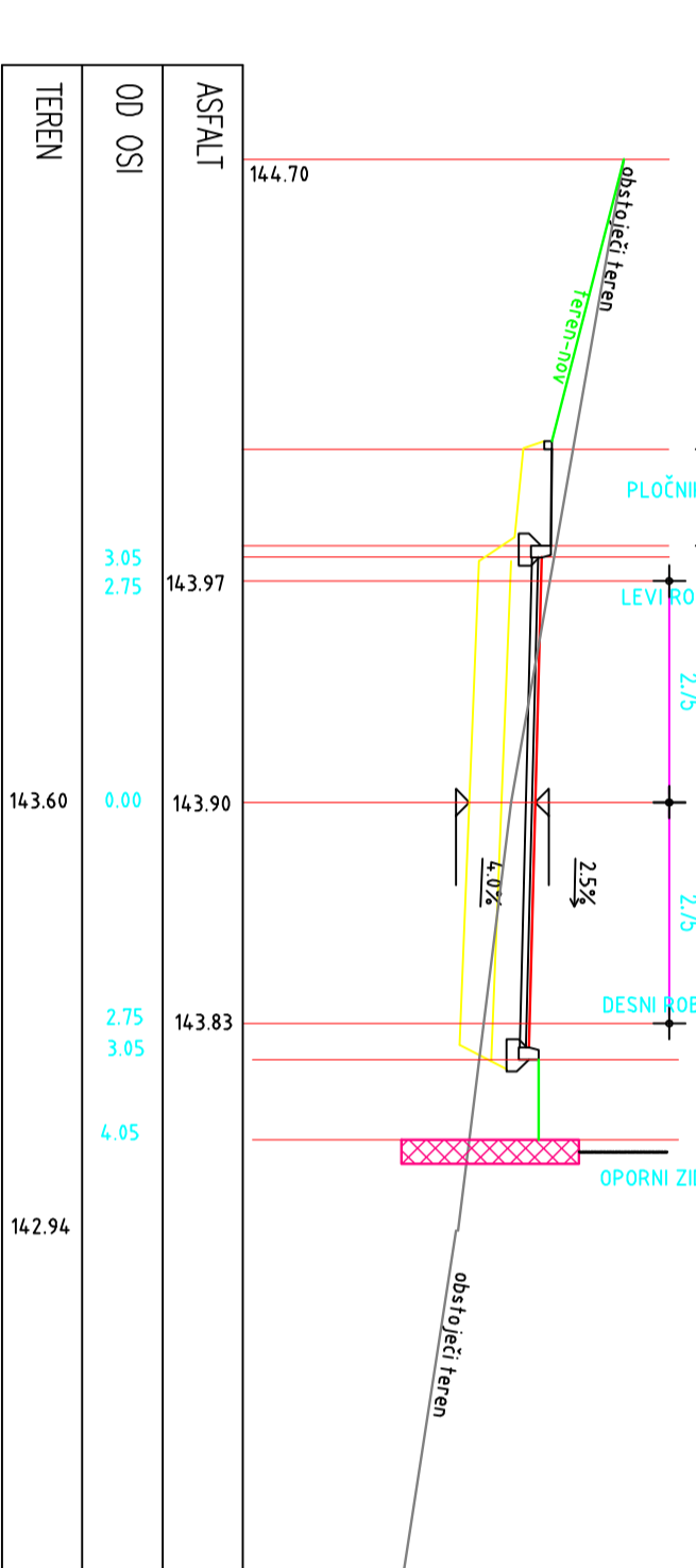
PREČNÍ PROFIL P7 0+070.00
