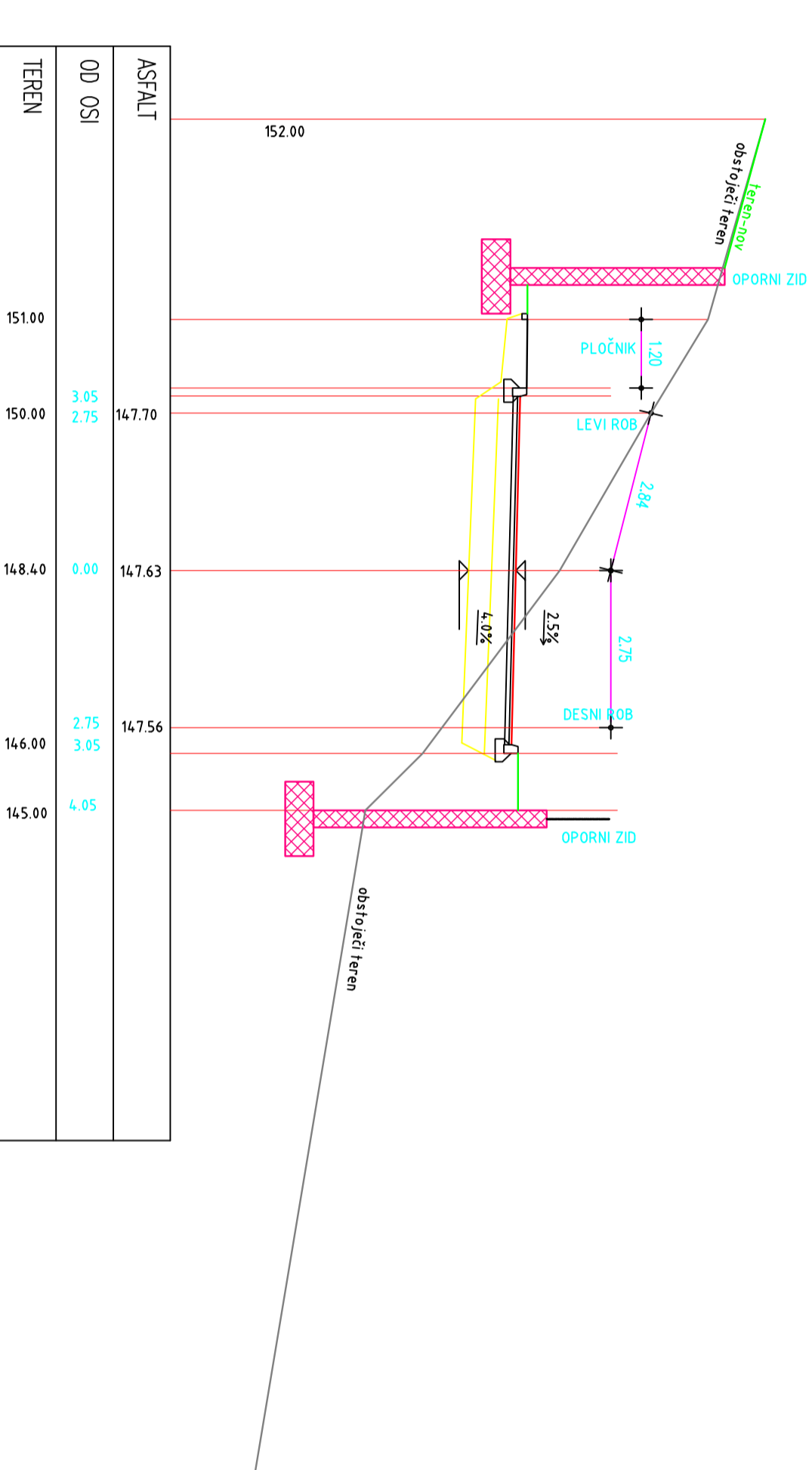
PREČNÍ PROFIL P9 0+090.00
