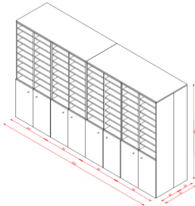
POGLED SPREDAJ
