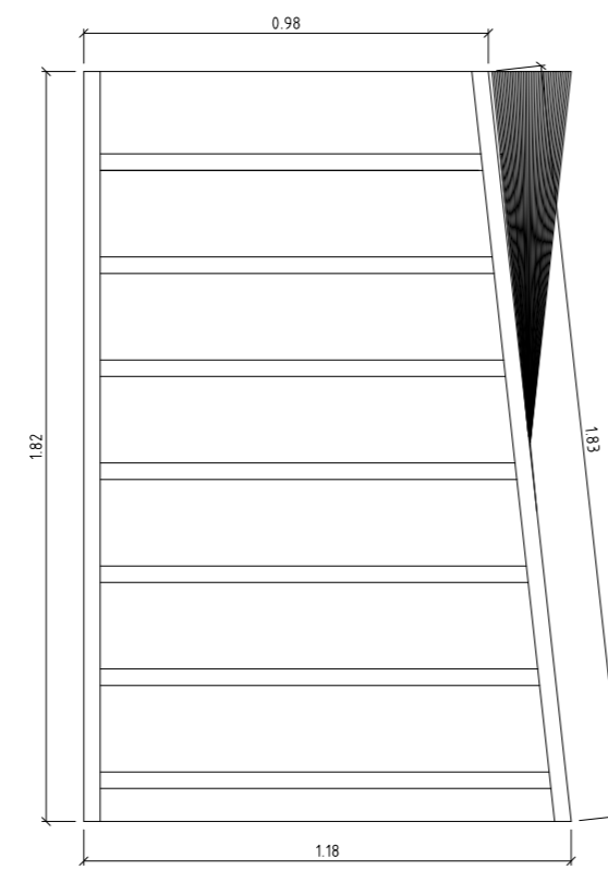
pograd - pogled 4 - M=1:20
