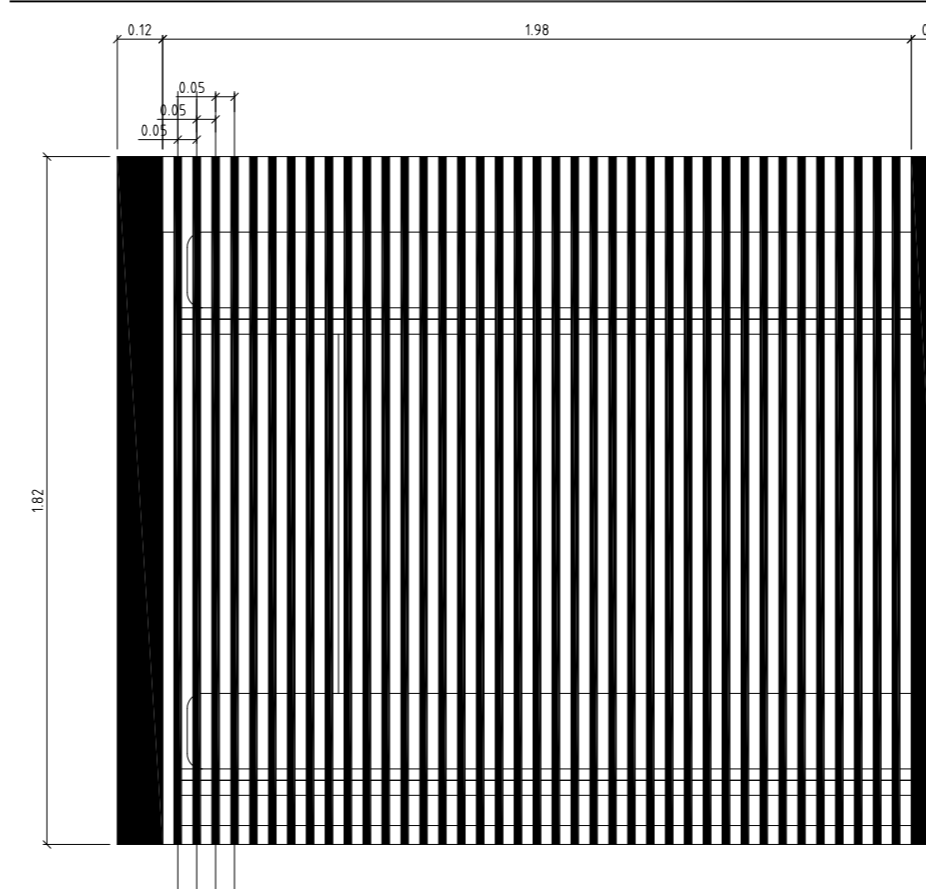
pograd - pogled 1 - M=1:20
