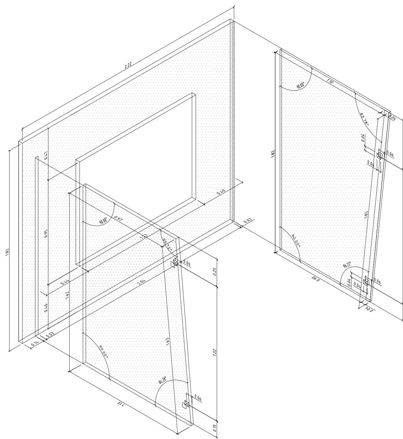
pograd - sestava obodnih plošč - M=1:20
