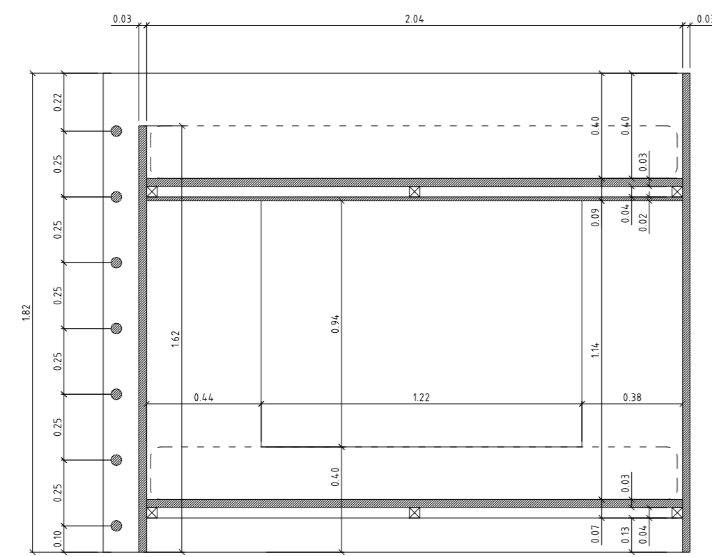
pograd - prerez A-A - M=1:20
