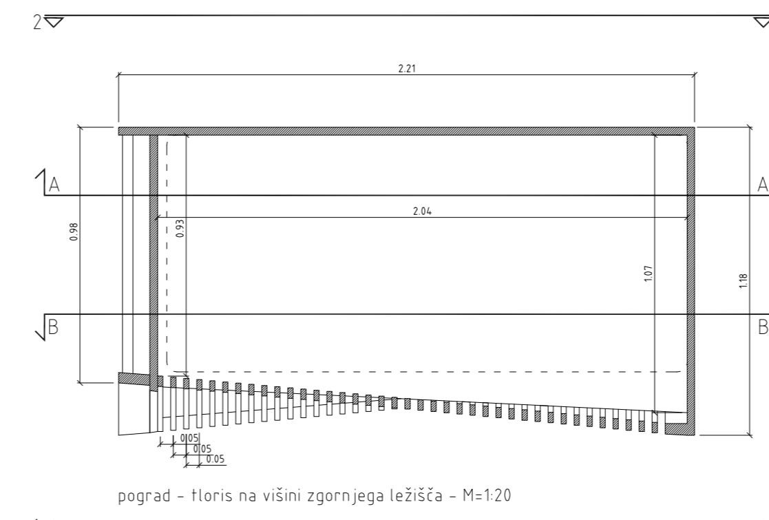
pograd - Floris na višini zgornjega ležišča - M=1:20
