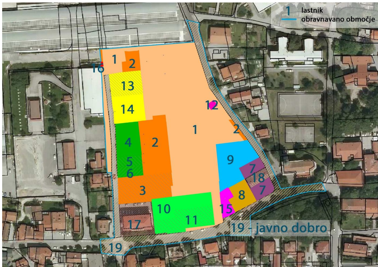
Slika 13: Prikaz lastništva
